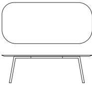
7SEL104 L240 P110 H74
